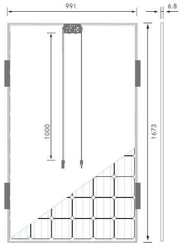
Rück-/ Vorder-/Seitenansicht 3
