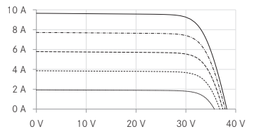
UI-Kennlinie Bsp. LX-280M/156-60+ GG
