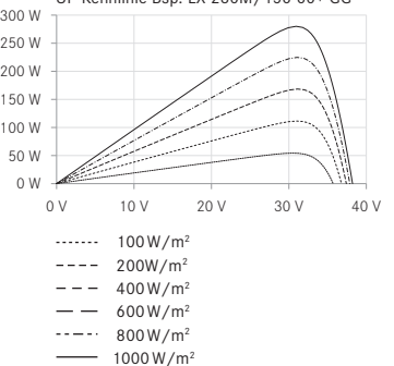
UP-Kennlinie Bsp. LX-280M/156-60+ GG
